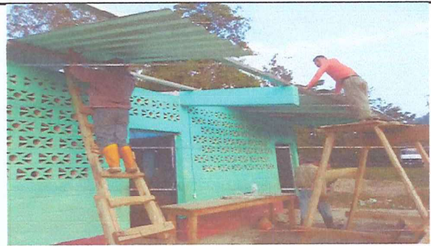
Foto 4: Se observa el reemplazo de estructura de techo del edificio de 4 aulas y dirección. (11-11-2024).
